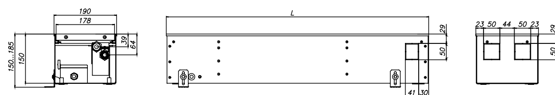
ЕКQ.190.150, вид сбоку
