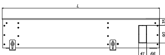
ЕКН.240.200, вид сбоку
