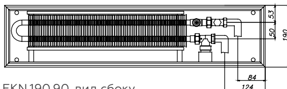
EKN.190.90, вид сбоку
