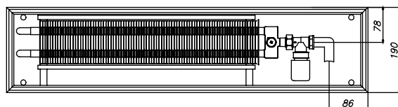
EKN.190.150, вид сбоку
