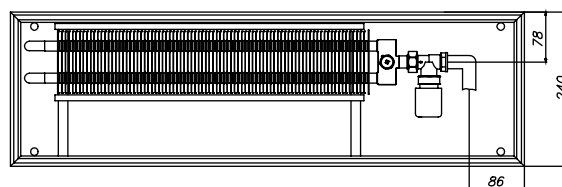
ЕКН.240.150, вид сбоку
