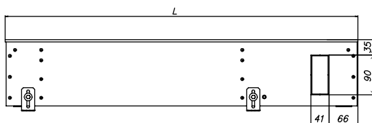
EKN.190.200, вид сбоку
