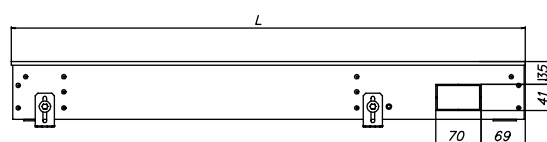
ЕКН.240.120, вид сбоку
