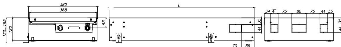
EKN.380.120, вид сбоку
