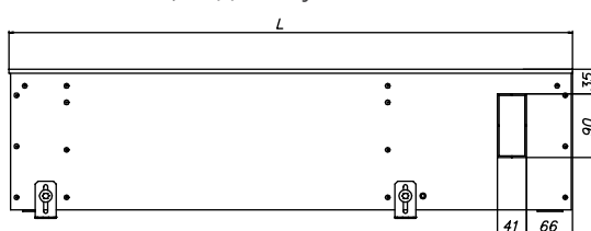
ЕКН.240.200, вид сбоку
