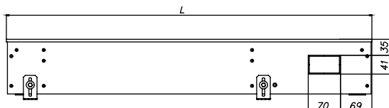
EKN.190.120, вид сбоку
