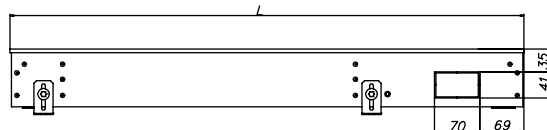
EKN.190.120, вид сбоку
