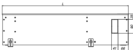
EKN.190.200, вид сбоку
