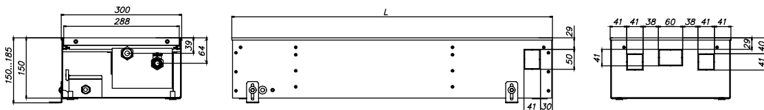
EKQ.300.150, вид сбоку
