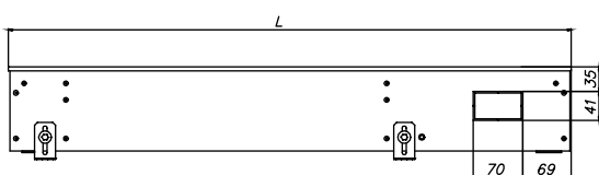
ЕКН.240.120, вид сбоку
