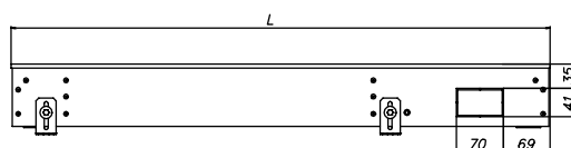
EKN.300.120, вид сбоку
