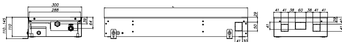
EKQ.300.110, вид сбоку
